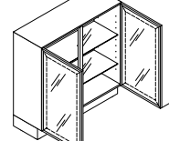
UDDDS Base unit with glass door DS ↔ 80/90/100 ↑ 90 ↙ 35
