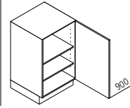
UDD Base unit ↔ 30/35/40/45/50/60 ↑ 90 ↙ 60/35
