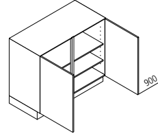
UDD Base unit ↔ 80/90/100/120 ↑ 90 ↙ 60/35
