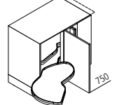
UELAD Corner base unit „LE MANS“ ↔ 110/115/125 ↑ 75 ↙ 60
