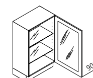
UDDDE Base unit with glass door DE ↔ 40/45/50/60 ↑ 90 ↙ 35
