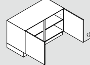
UDD Base unit ↔ 80/90/100/120 ↑ 60 ↙ 60/35
