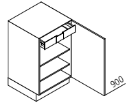
UDDI Base unit ↔ 40/45/50/60 ↑ 90 ↙ 60
